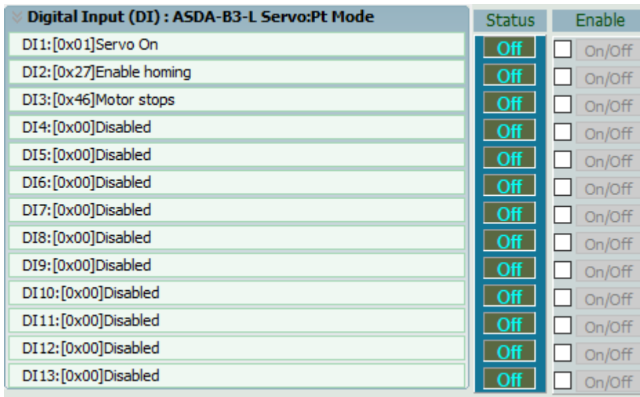
Рис. 7.1.5.2 Настройка DI/O в ПО ASDA-Soft
