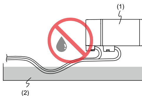
(1) Серводвигатель; (2) Масло
