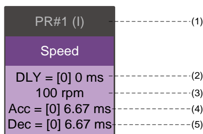
Рис. 7.1.4.3 Отображение команды скорости
