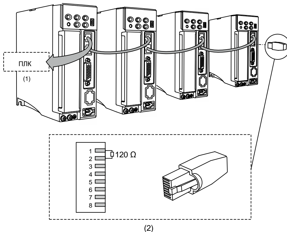
(1) Подключение ПЛК; (2) Подключение терминального резистора CAN
