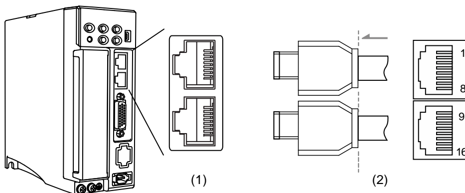
(1) Разъем CN3 (розетка); (2) разъем CN3 (штекер)
