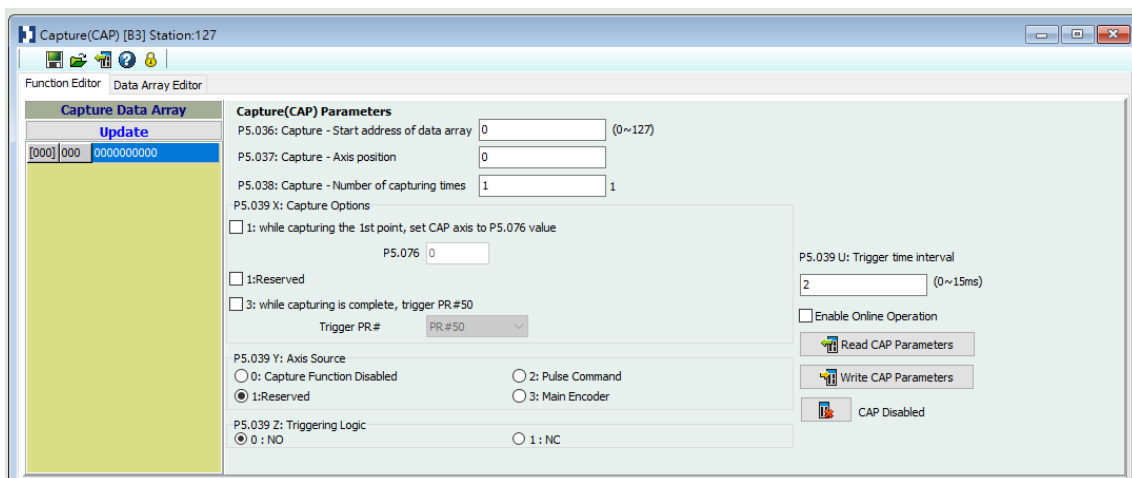
Рис. 7.2.2.2 Экран функции захвата в ПО ASDA-Soft
