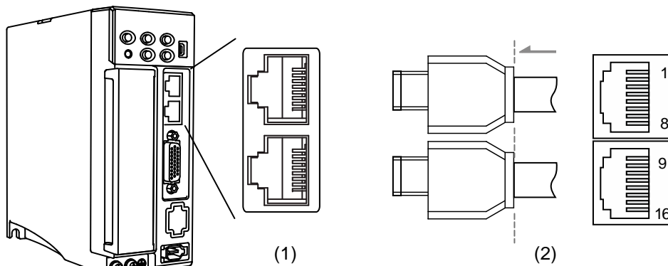
(1) Разъем CN6 (розетка); (2) Разъем CN6 (штекер)
